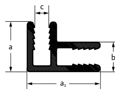
Eckverbindungsprofil
